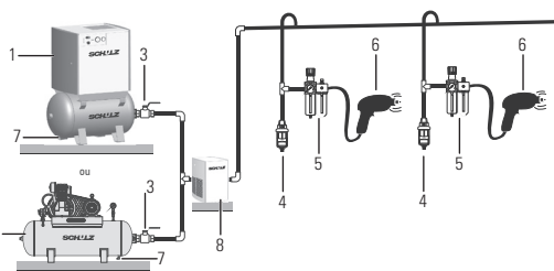
FIGURA 1 - ESQUEMA INSTALACIÓN ORIENTATIVO
