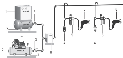
FIGURA 1 - ESQUEMA DE INSTALAÇÃO ORIENTATIVO
