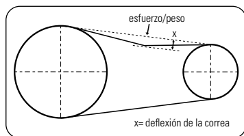
FIGURA 7.15 - DEFLEXIÓN DE LA CORREA
