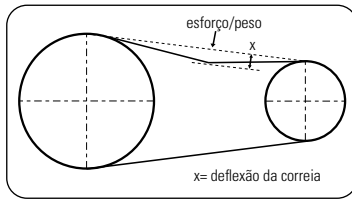
FIGURA 7.15 - DEFLEXÃO DA CORREIA
