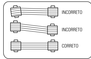
FIGURA 7.16 - ALINHAMENTO DA POLIA
