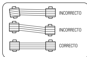
FIGURA 7.16 - ALINEAMIENTO DE LA POLEA
